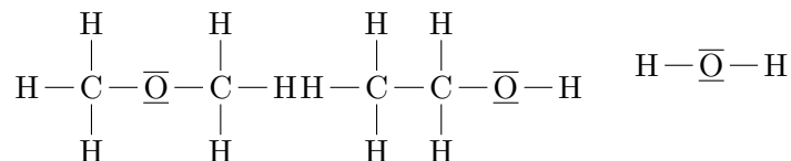
Méthoxyméthane
