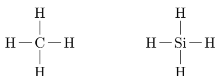
Méthane
